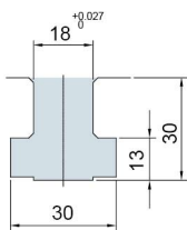
T-Slot
